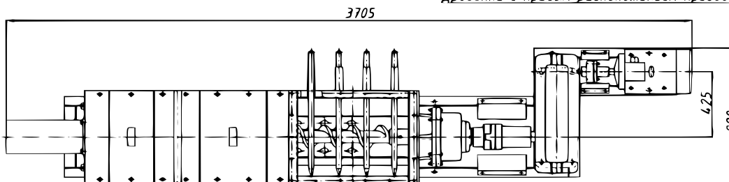
Дробилка с правым расположением привода
